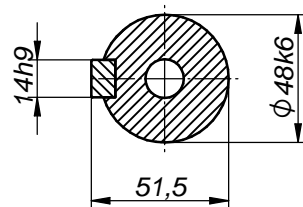
A-A (1:2)
